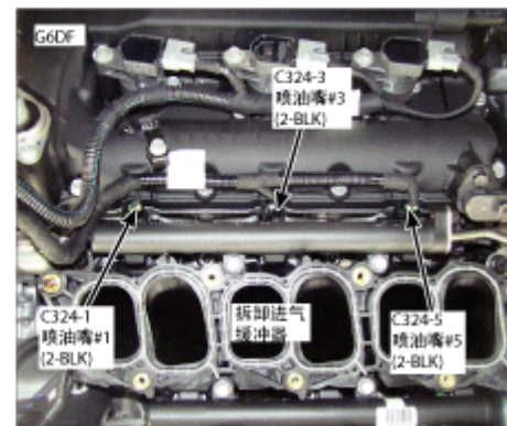
186.发动机顶部
