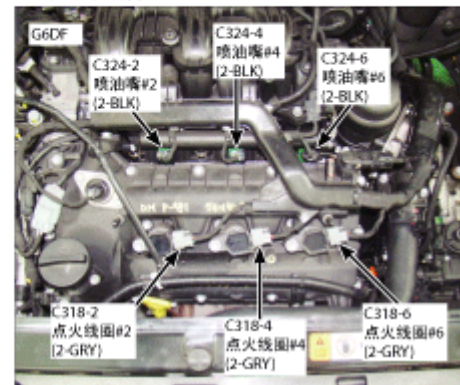
183.发动机顶部
