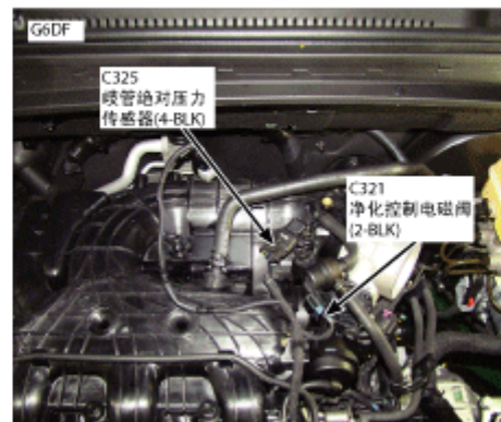
185.发动机顶部
