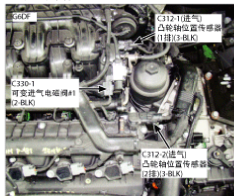
184.发动机后部
